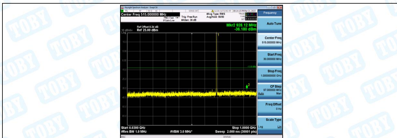
Band12-1.4MHz-QPSK-23017-1-0-Low-30-1000--36.18-PASS
