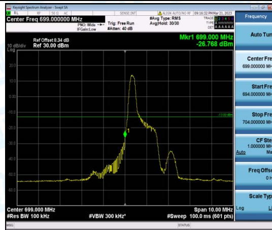
Band12-5MHz-QPSK-23035-1-0-Low--26.77-PASS
