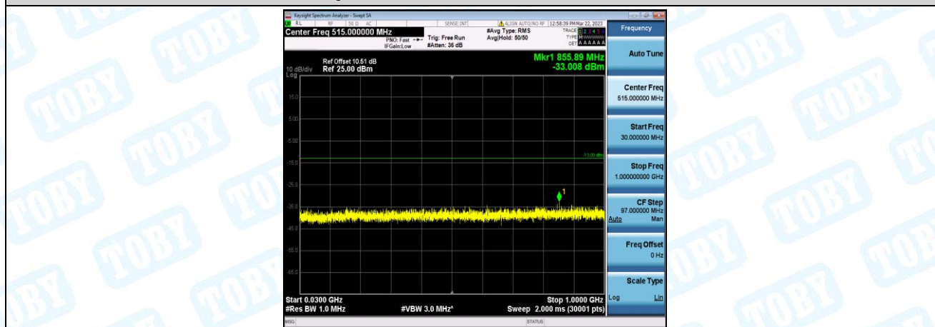
Band66-10MHz-QPSK-132322-1-0-Low-30-1000--33.01-PASS
