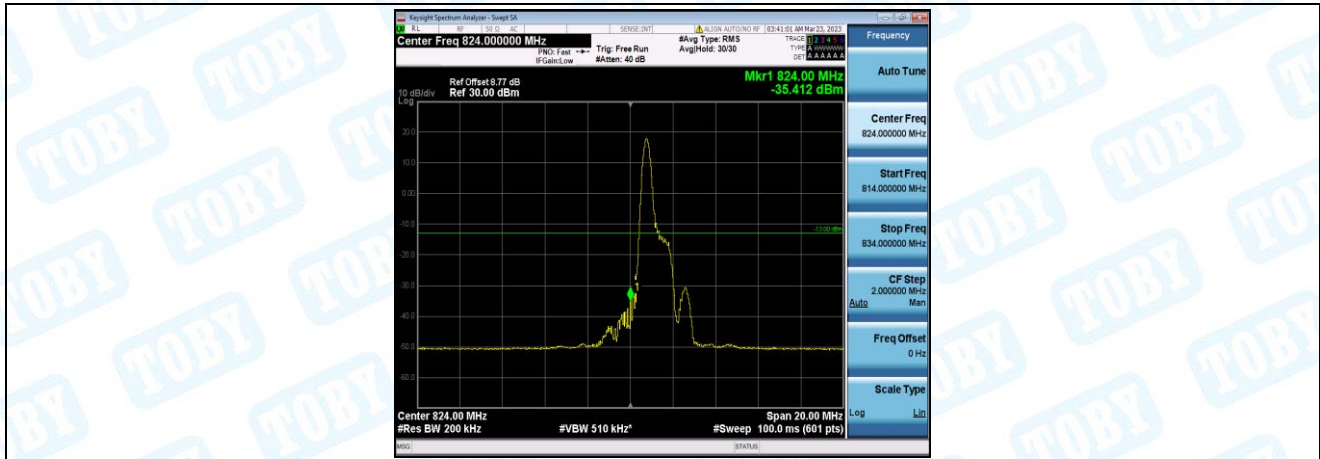
Band26-10MHz-QPSK-26840-1-0-Low--35.41-PASS
