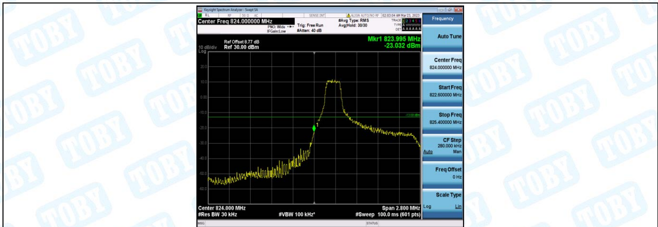
Band26-1.4MHz-QPSK-26797-1-0-Low--23.03-PASS
