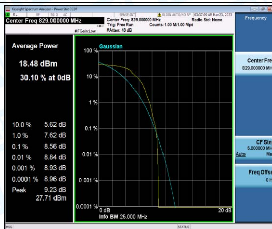
Band26-10MHz-QPSK-26840-1-0-Low-8.56-=<13-PASS
