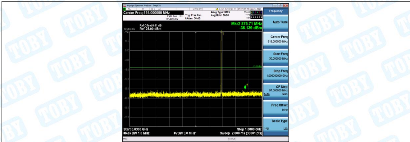
Band12-10MHz-16QAM-23060-1-0-Low-30-1000--36.14-PASS
