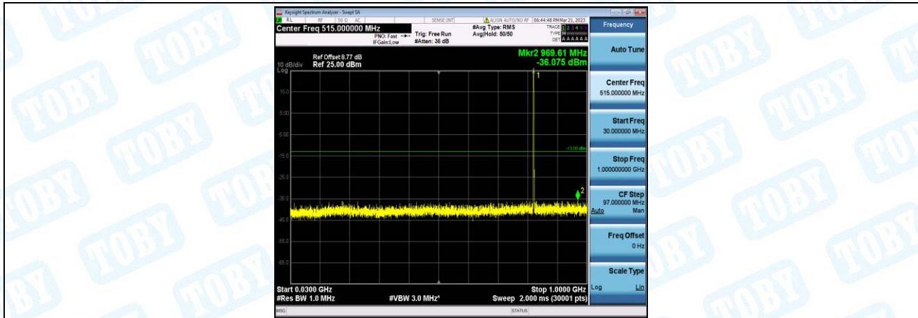
Band5-3MHz-16QAM-20415-1-0-Low-30-1000--36.08-PASS
