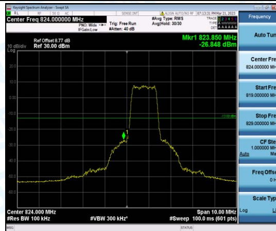
Band5-5MHz-QPSK-20425-6-0-Low--26.85-PASS
