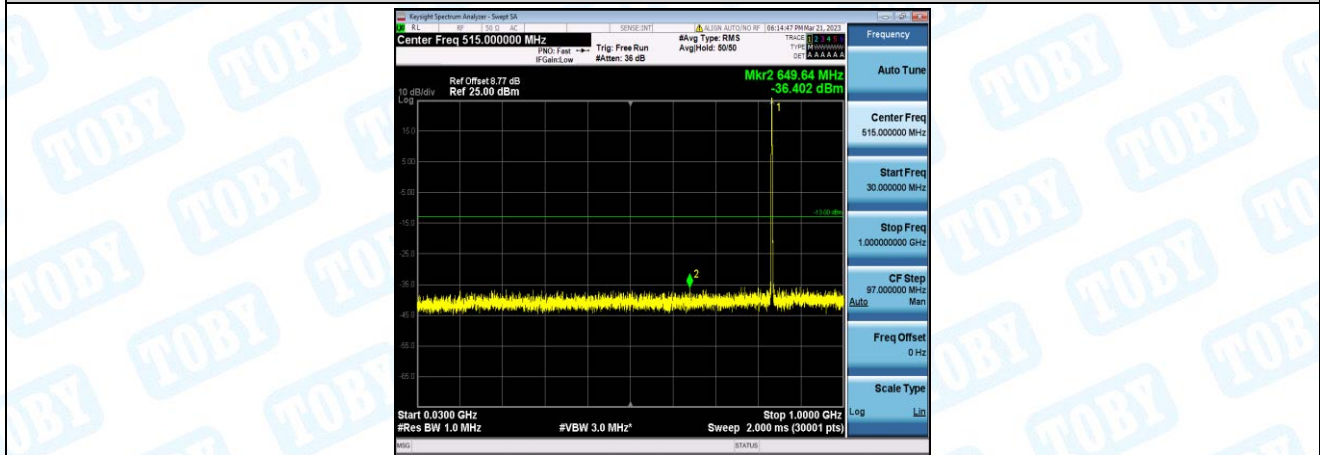
Band5-1.4MHz-QPSK-20525-1-0-Low-30-1000--36.4-PASS
