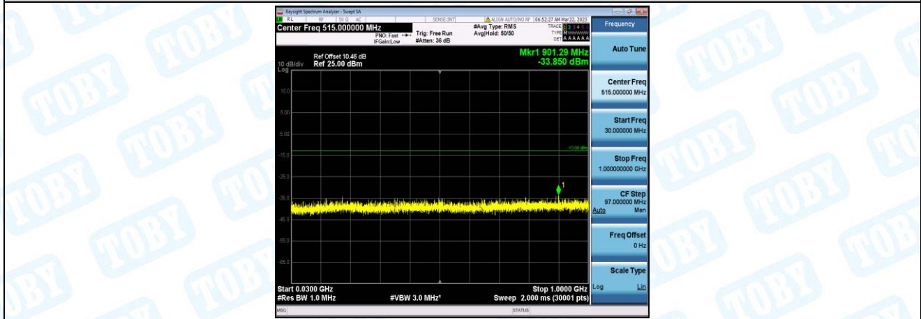
Band4-5MHz-QPSK-20175-1-0-Low-30-1000--33.85-PASS
