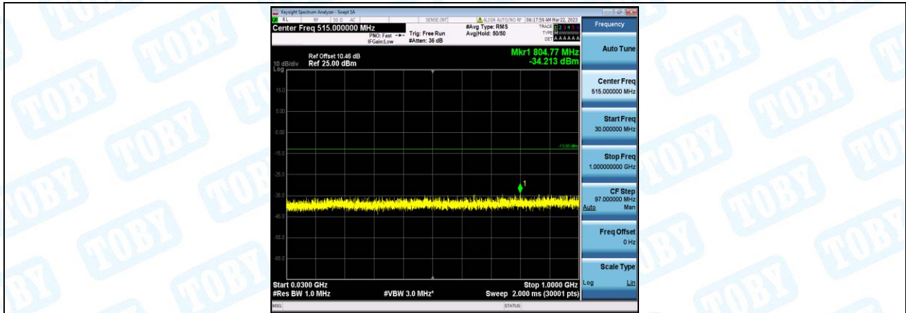
Band4-3MHz-QPSK-19965-1-0-Low-30-1000--34.21-PASS
