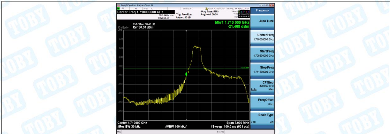
Band4-1.4MHz-QPSK-19957-1-0-Low--21.47-PASS
