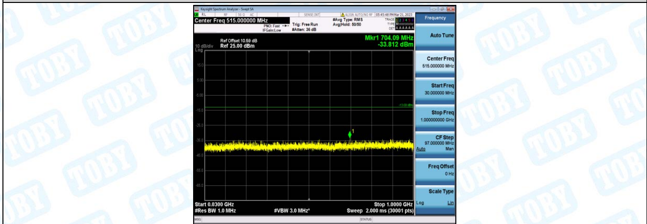
Band2-20MHz-QPSK-18900-1-0-Low-30-1000--33.81-PASS
