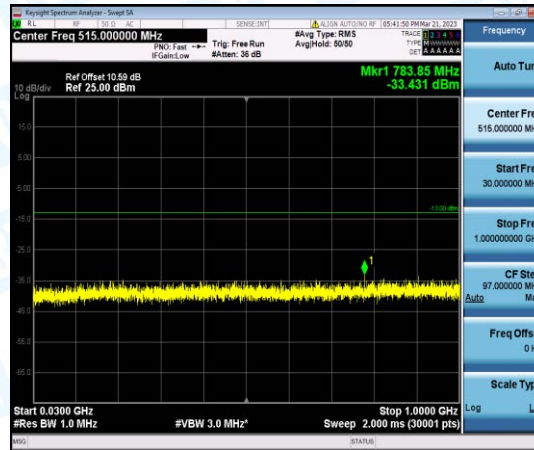
Band2-20MHz-QPSK-18700-1-0-Low-30-1000--33.43-PASS
