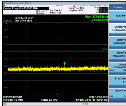
Band2-10MHz-QPSK-18650-1-0-Low-30-1000--33.81-PASS
