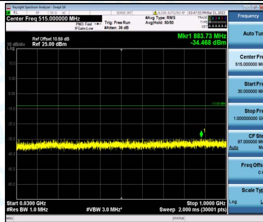
Band2-3MHz-QPSK-18900-1-0-Low-30-1000--34.47-PASS
