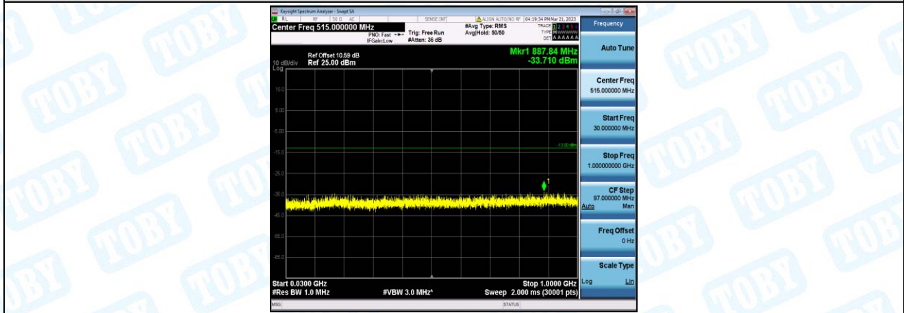
Band2-5MHz-QPSK-18900-1-0-Low-30-1000--33.71-PASS
