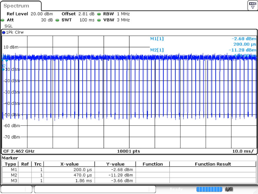
Test_Graph_802.11g_ANT1_2462
