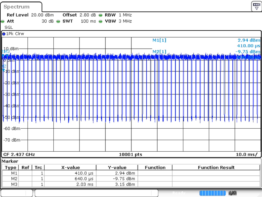
Test_Graph_802.11g_ANT1_2437
