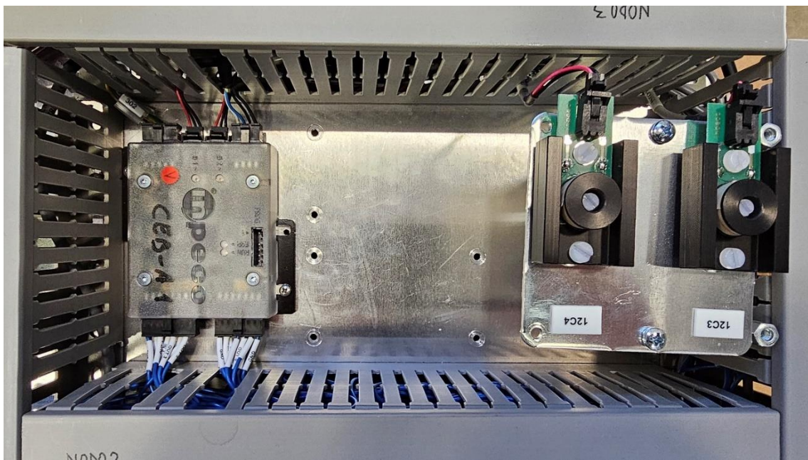
EUT + Antennas
