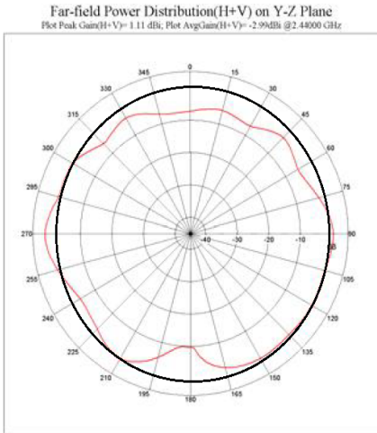
YZ-plane
