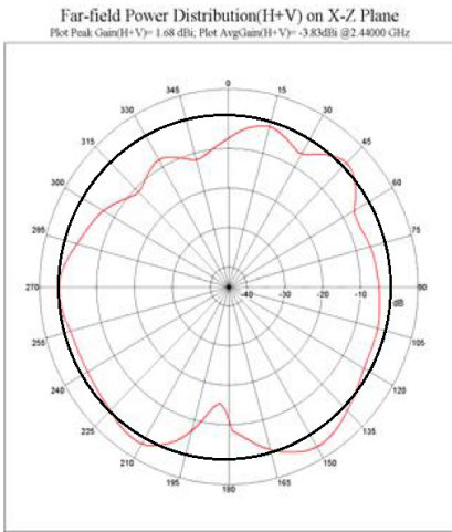
XZ-plane
