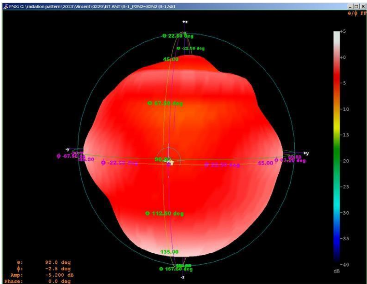
XY-plane
