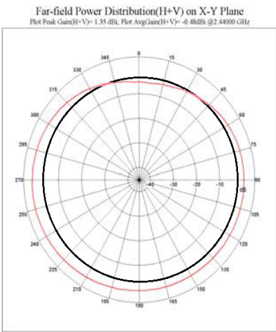
XY-plane
