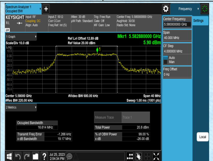
11A-Ant1-5580
