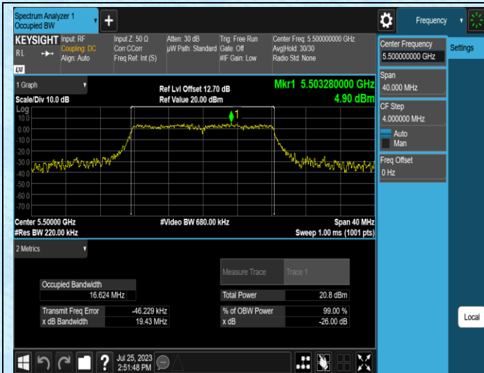
11A-Ant1-5500
