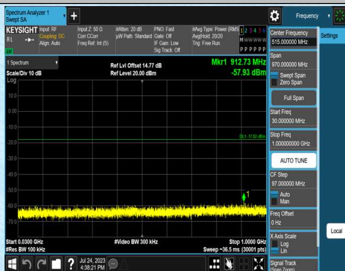
2DH5-Ant1-2402-30~1000
