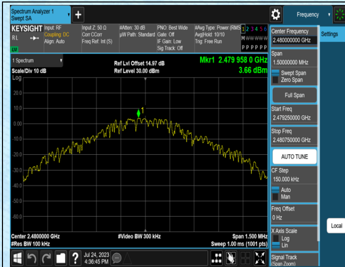
DH5-Ant1-2480-0-Reference
