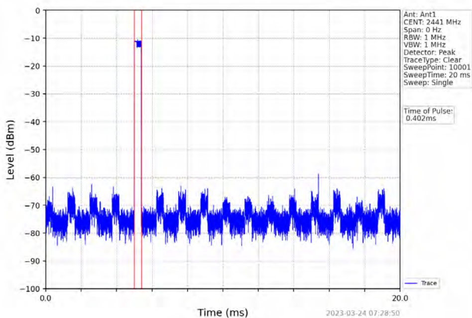
Pi/4DQPSK 2DH1_HOPP
