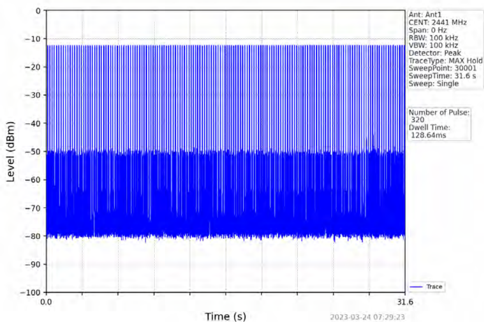
Pi/4DQPSK 2DH1_HOPP
