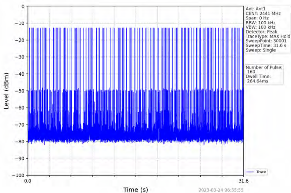
Pi/4DQPSK 2DH3 HOPP
