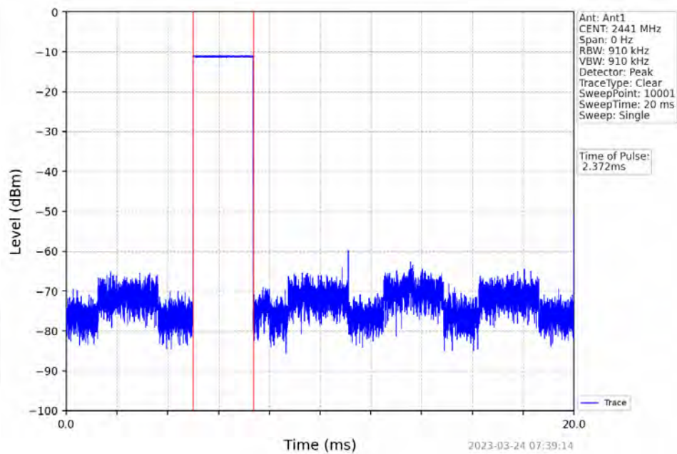
8DPSK 3DH5_HOPP
