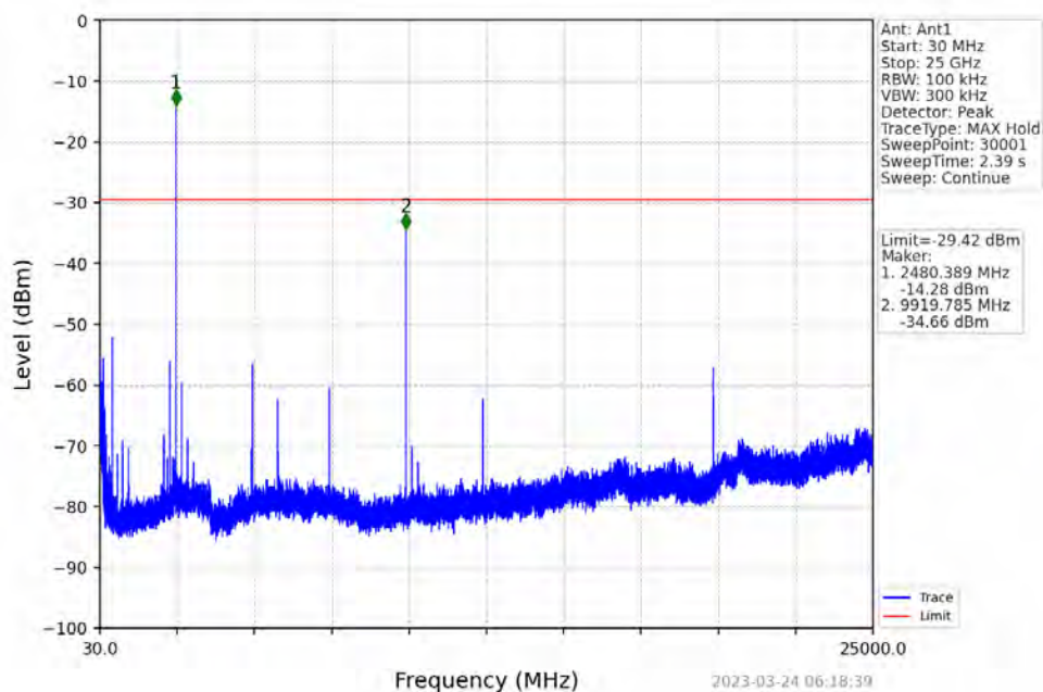
GFSK DH5 HOPP
