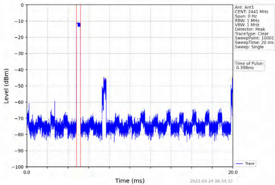
Pi/4DQPSK 2DH1_HOPP
