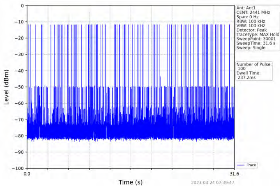
8DPSK 3DH5_HOPP
