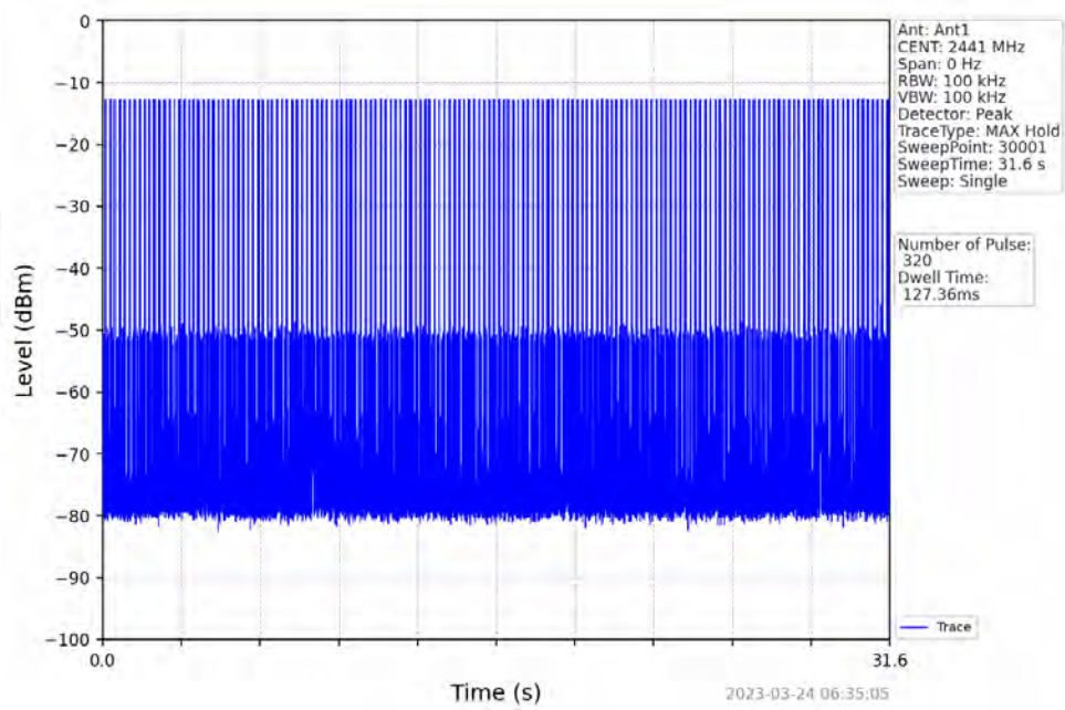
Pi/4DQPSK 2DH1_HOPP
