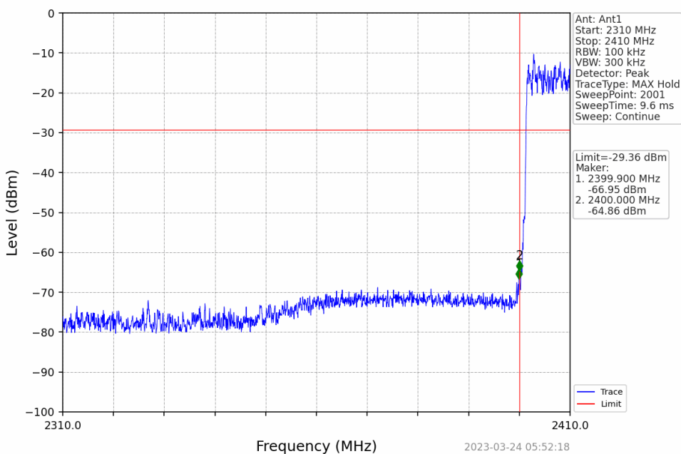
Pi/4DQPSK_2DH5_HOPP
