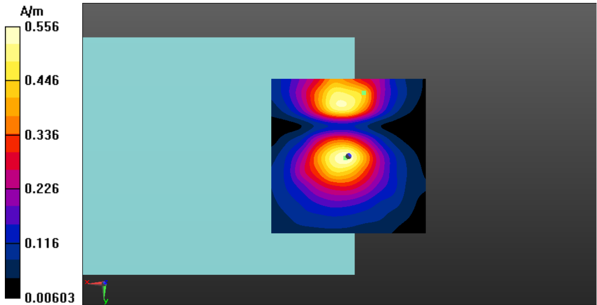
Fig A.18 T-Coil WCDMA Band 2-Y
