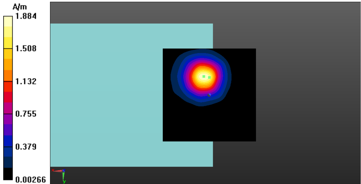
Fig A.17 T-Coil EDGE 850-Z
