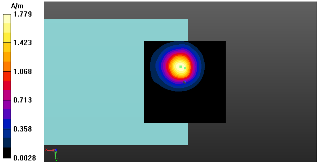
Fig A.18 T-Coil WCDMA Band 2-Z
