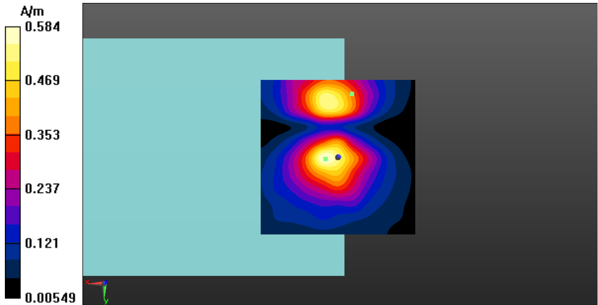
Fig A.17 T-Coil EDGE 850-Y
