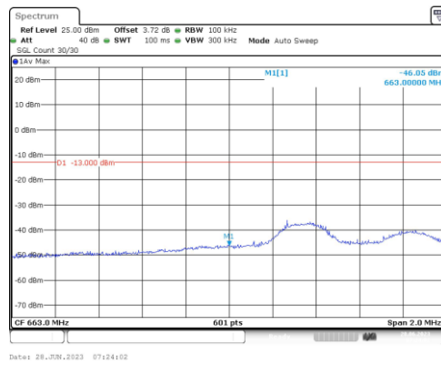
Band71-5MHz-QPSK-133147-1RB#24
