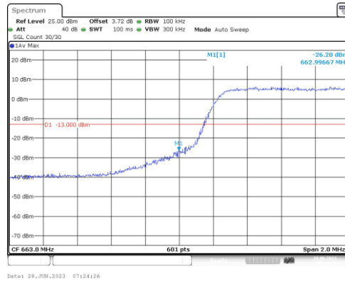
Band71-5MHz-QPSK-133147-25RB#0
