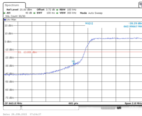
Band71-5MHz-QPSK-133147-25RB#0
