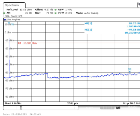
Band66-20MHz-QPSK-132072-1RB#0-Range4:1000~20000MHz
