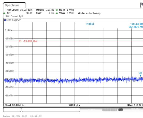
Band66-20MHz-QPSK-132072-1RB#0-Range3:30~1000MHz
