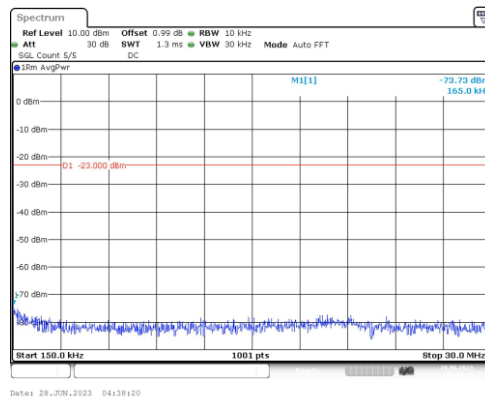
Band66-3MHz-QPSK-131987-1RB#0-Range2:0.15~30MHz
