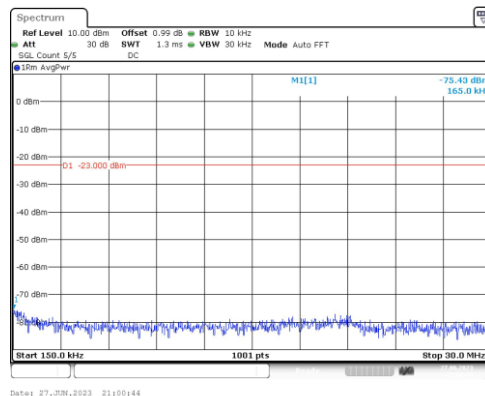
Band4-3MHz-QPSK-19965-1RB#0-Range2:0.15~30MHz
