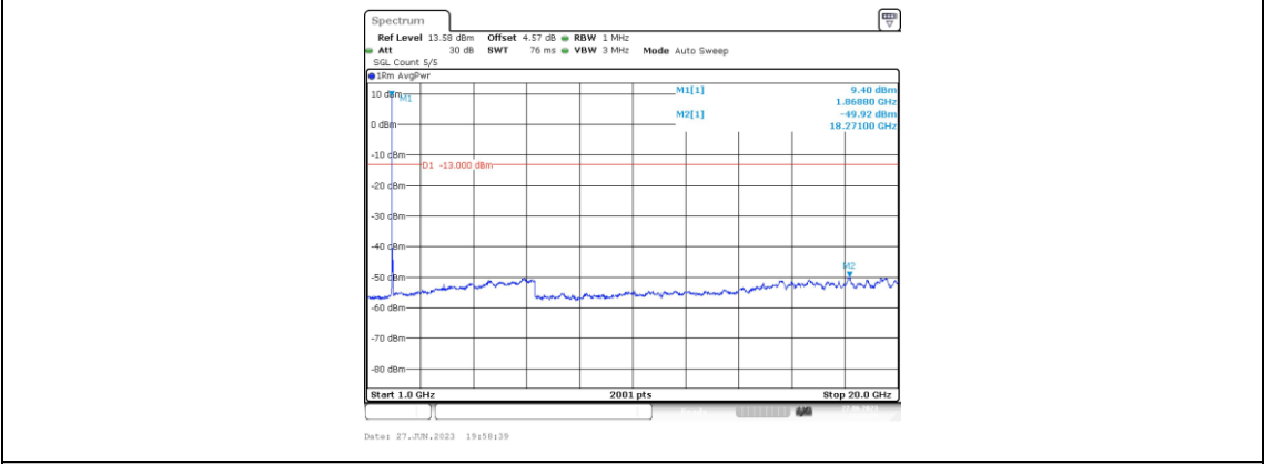
Band2-20MHz-QPSK-18900-1RB#0-Range4:1000~20000MHz
