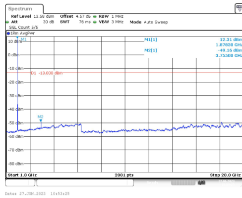
Band2-5MHz-QPSK-18900-1RB#0-Range4:1000~20000MHz
