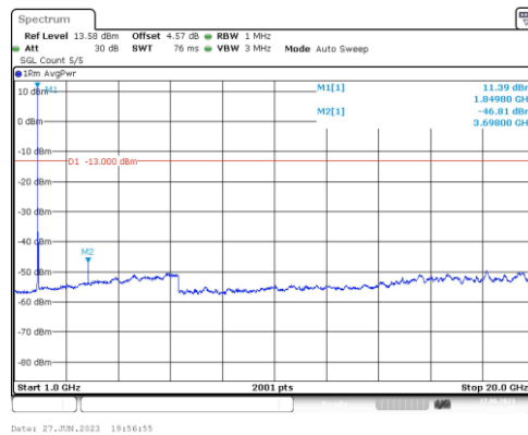
Band2-20MHz-QPSK-18700-1RB#0-Range4:1000~20000MHz
