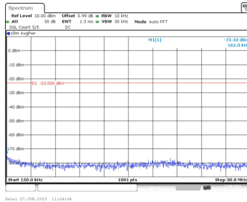
Band2-10MHz-QPSK-18900-1RB#0-Range2:0.15~30MHz
