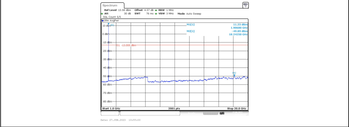
Band2-5MHz-QPSK-19175-1RB#0-Range4:1000~20000MHz
