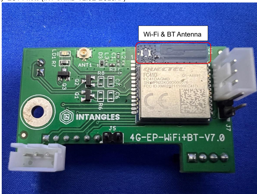
(8) EUT Photo (INT-SHMD-V2.0E-EC25AF)
