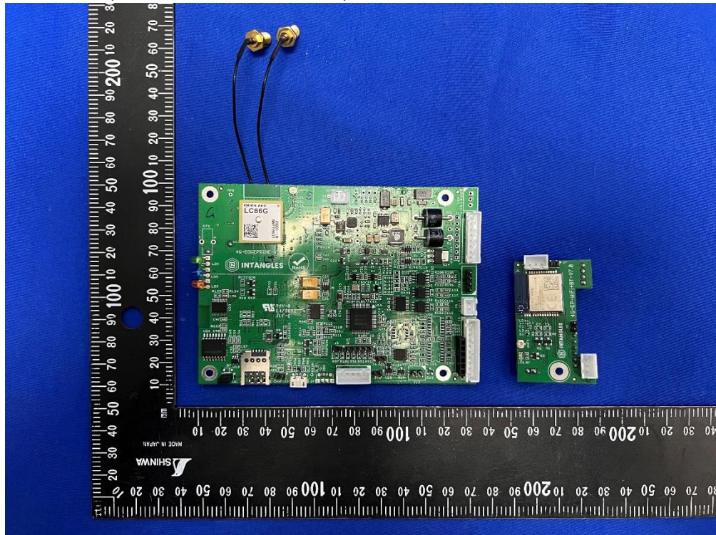
(2) EUT Photo (INT-SHMD-V2.0E-EC25AF)
