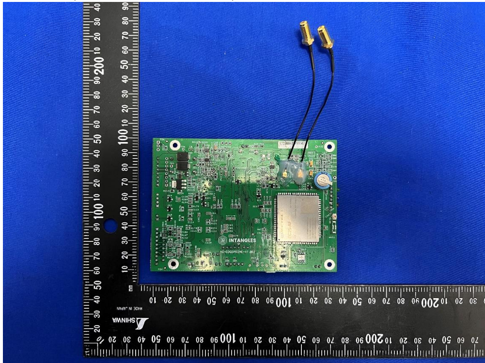
(3) EUT Photo (INT-SHMD-V2.0E-EC25AF)
