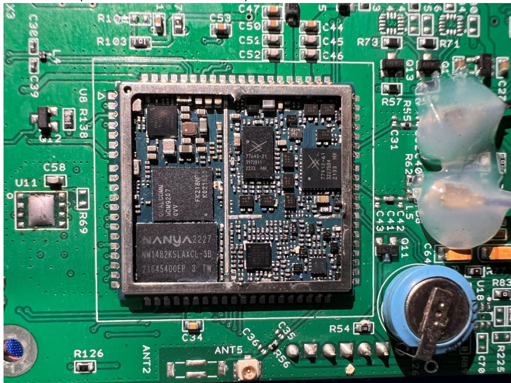
(5) EUT Photo (INT-SHMD-V2.0E-EC25AF)
