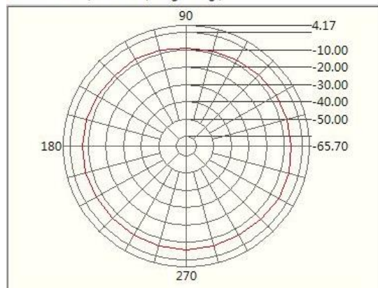
4.8GHz@Theta
