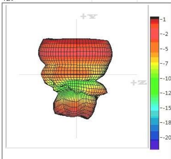
4.8GHzRight-Left
