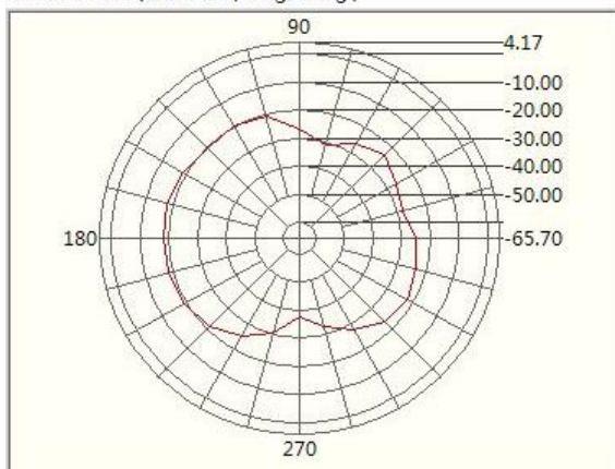
4.8GHzRight-Left
