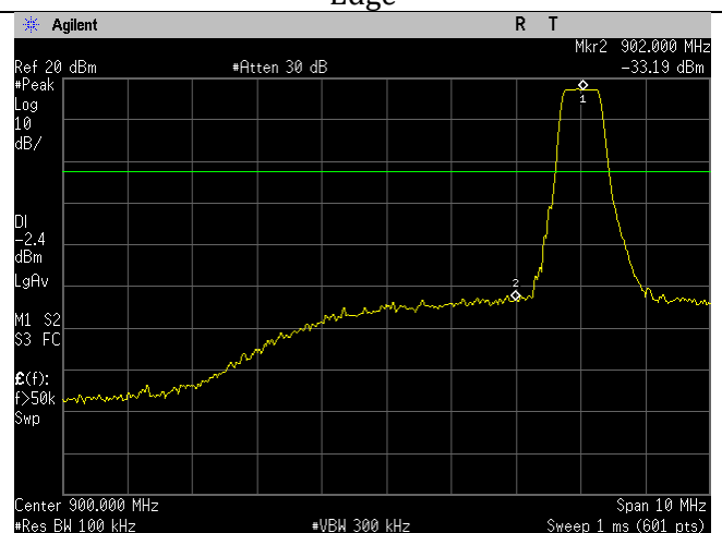
Low Ch_903MHz_500kHz_20dBc_Lower Band Edge
