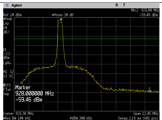
High Ch_914.2MHz_500kHz_20dBc_Upper Band Edge
