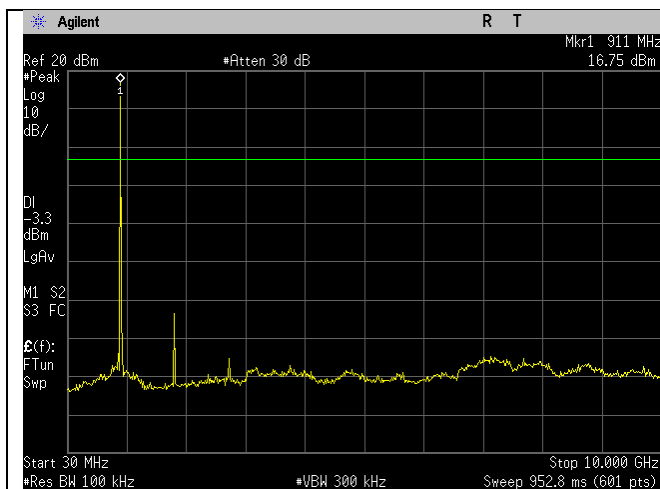
High Ch_914.2MHz_500kHz_20dBc_30MHz-10GHz
