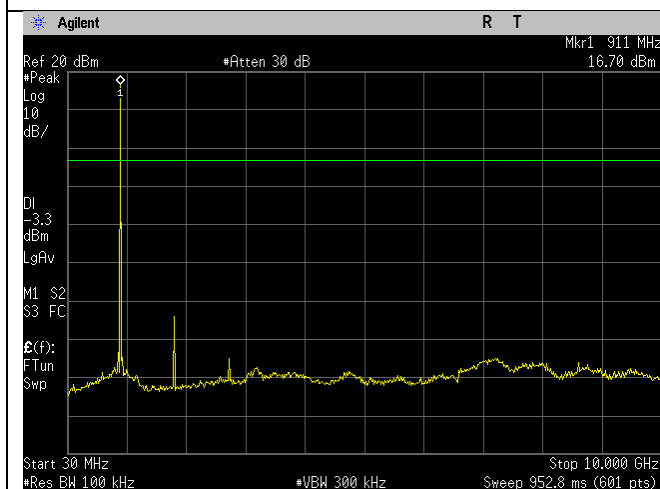
Low Ch_902.3MHz_125kHz_20dBc_30MHz-10GHz
