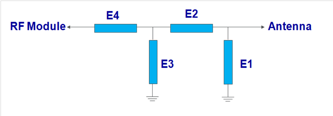
匹配电路 matching circuit
