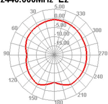
2440.000MHz E2
