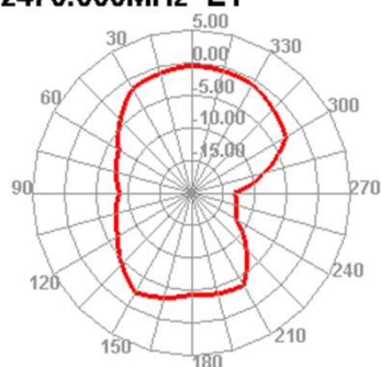
2470.000MHz E1
