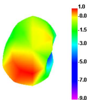
2490.000MHz E1
