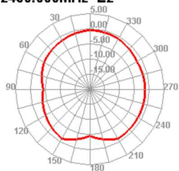
2450.000MHz E2
