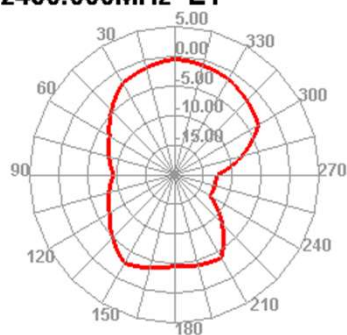
2450.000MHz E1
