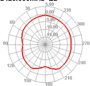
2420.000MHz E2
