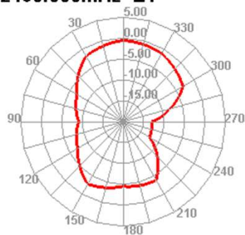
2460.000MHz E1
