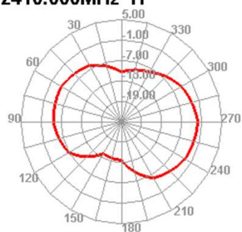
2410.000MHz H
