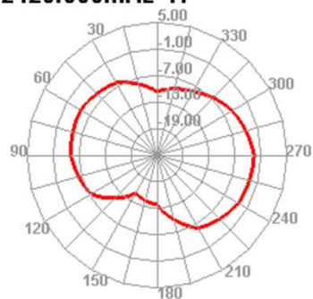
2420.000MHz H
