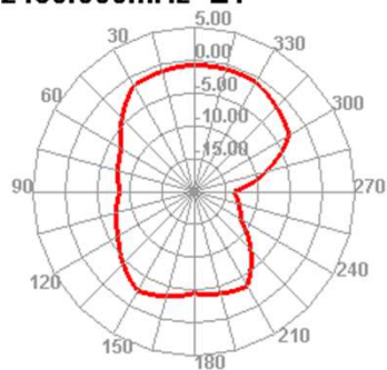
2480.000MHz E1
