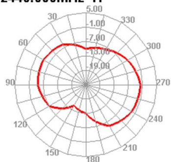
2440.000MHz H
