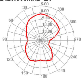
2420.000MHz E1
