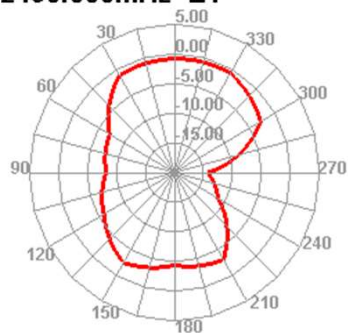
2490.000MHz E1
