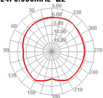
2470.000MHz E2
