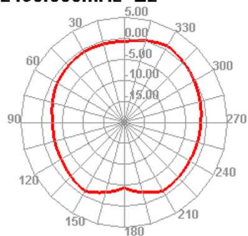
2490.000MHz E2
