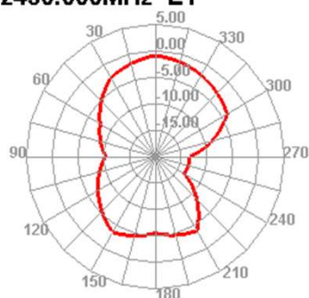
2430.000MHz E1
