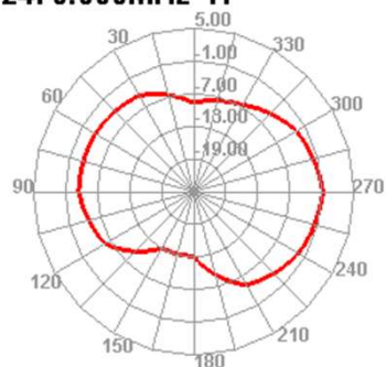
2470.000MHz H
