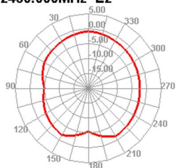
2430.000MHz E2
