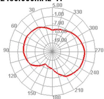
2430.000MHz H
