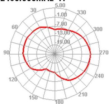
2460.000MHz H
