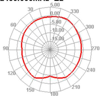
2480.000MHz E2
