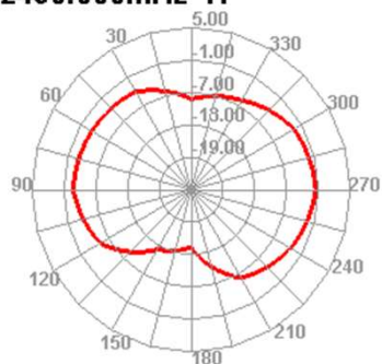
2490.000MHz H
