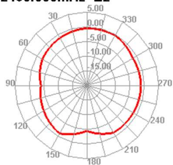
2460.000MHz E2
