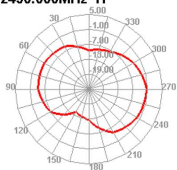
2450.000MHz H
