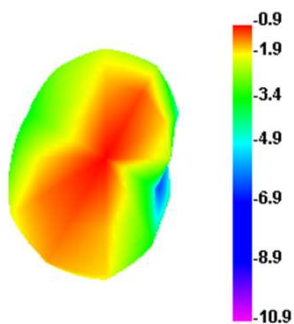
2420.000MHz
