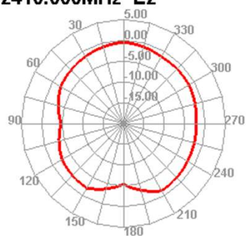
2410.000MHz E2
