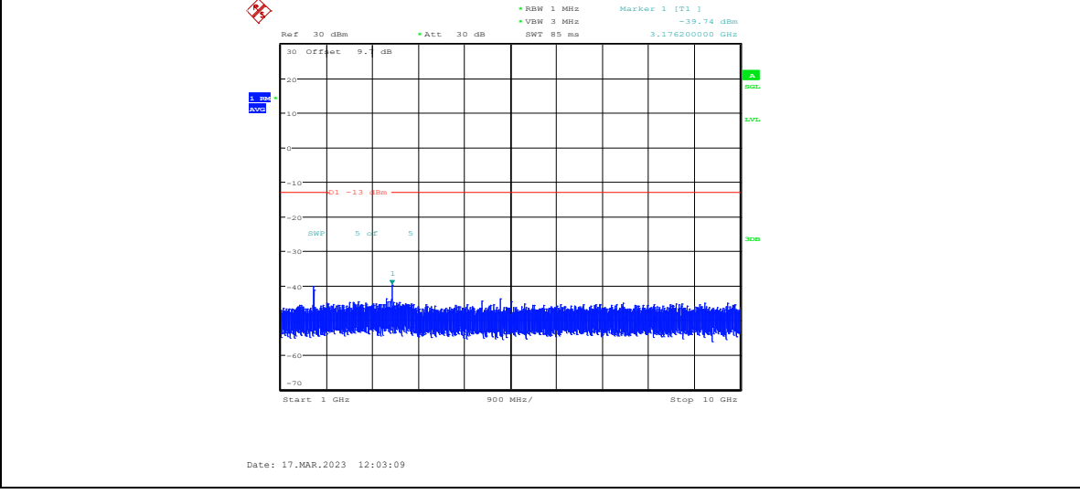
Band5-3MHz-QPSK-20415-1RB#0-Range4:1000~10000MHz
