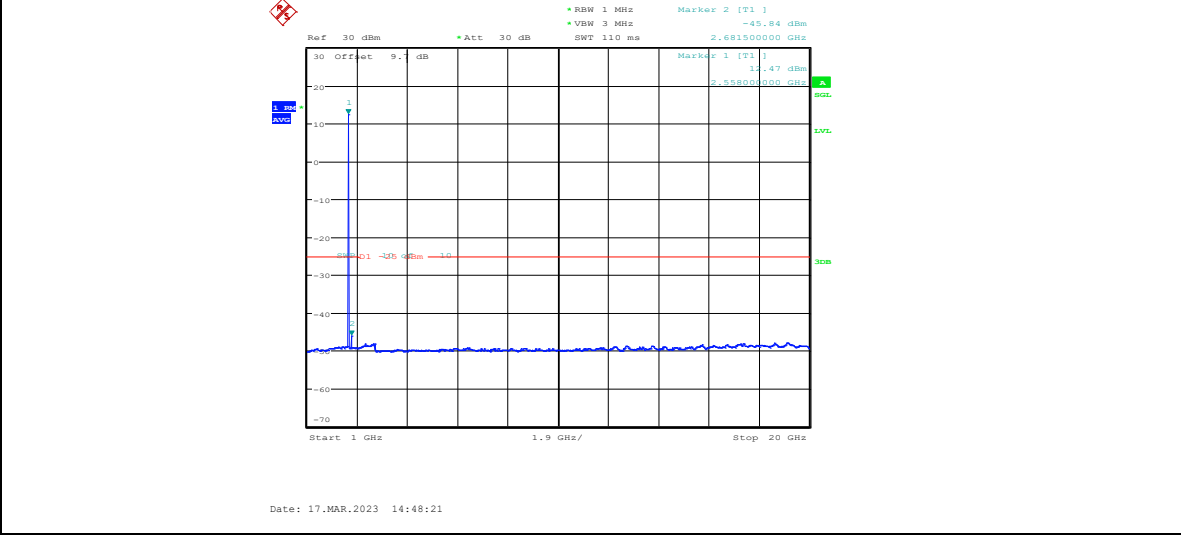
Band7-5MHz-QPSK-21425-1RB#0-Range4:1000~20000MHz
