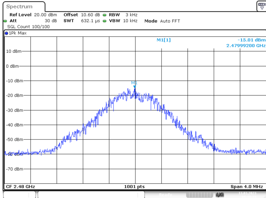
PSD NVNT 2M 2480MHz Ant1
