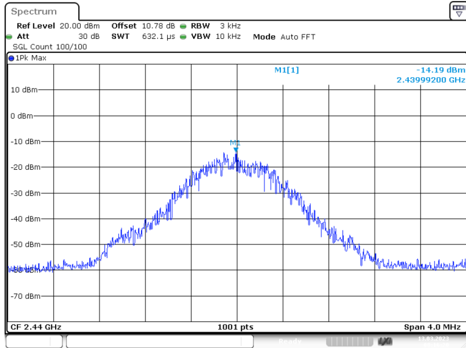
PSD NVNT 2M 2440MHz Ant1
