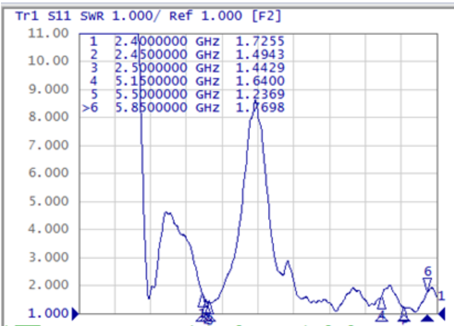
图 5 天线驻波
