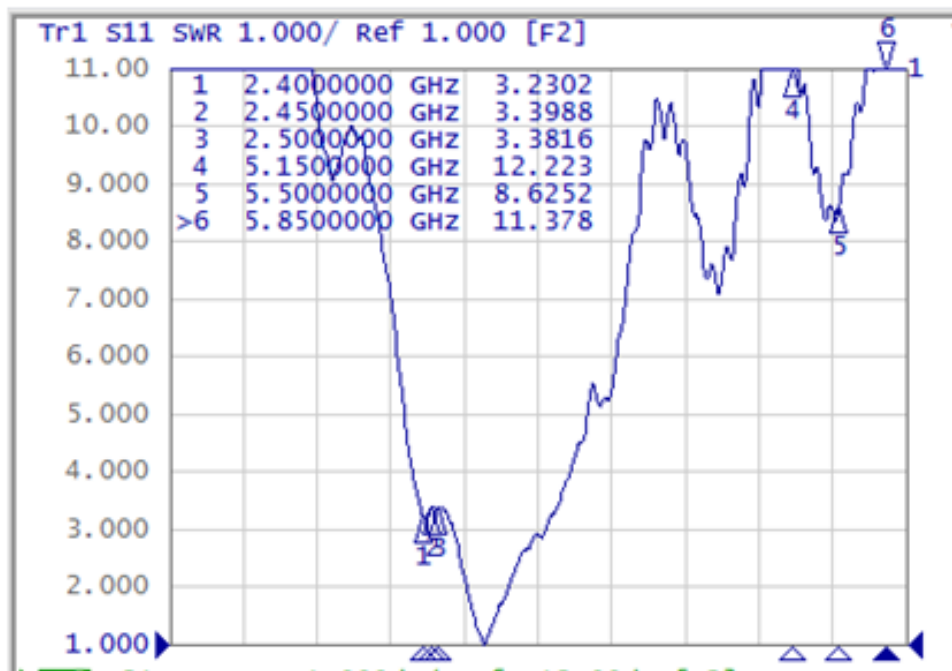
图 5 天线驻波
