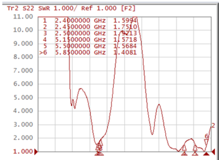
天线驻波图
