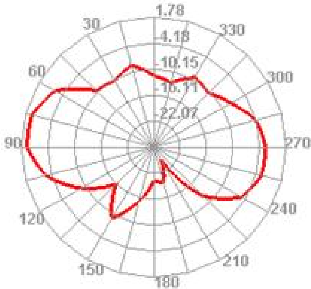
2450.000MHz E1
