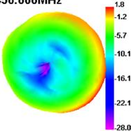
2450.000MHz E1
