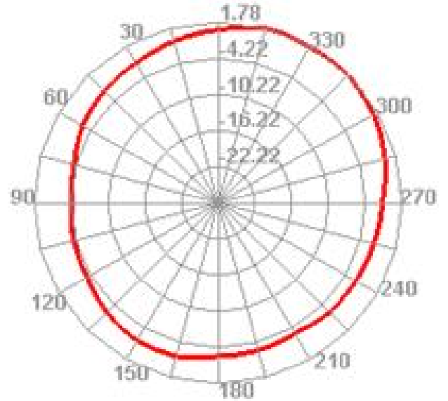
2450.000MHz H
