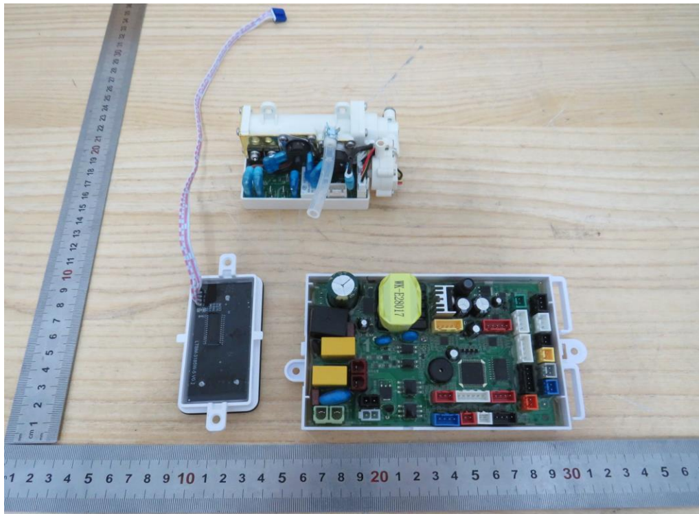
(3) EUT Photo
