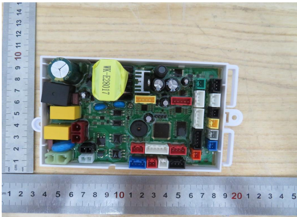
(4) EUT Photo
