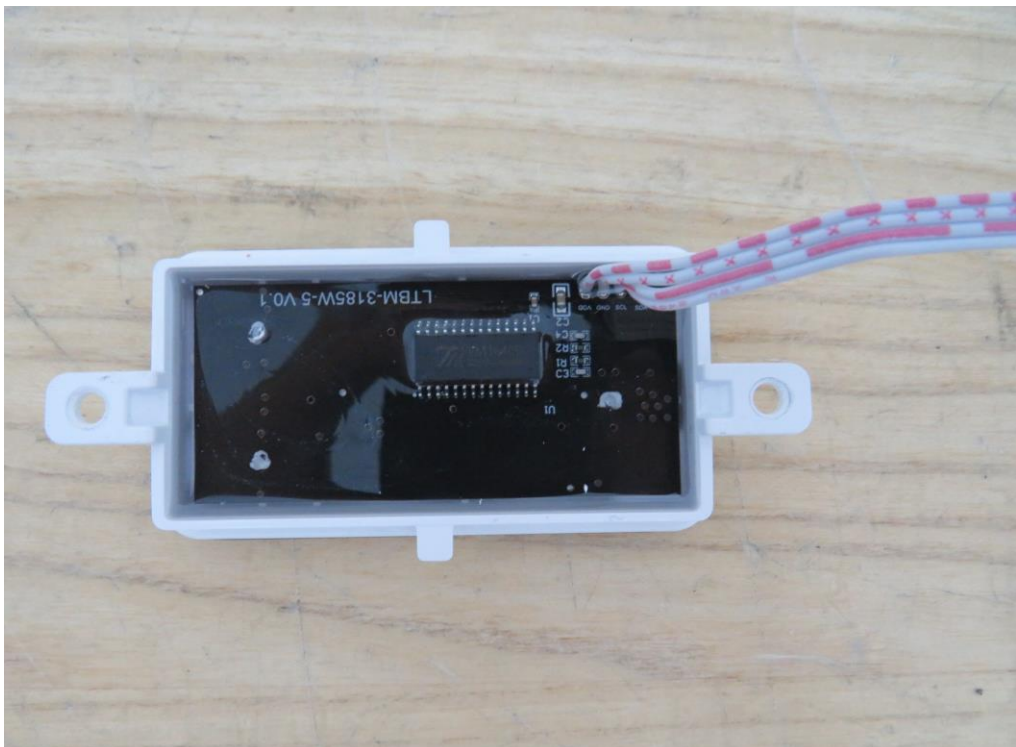
(8) EUT Photo
