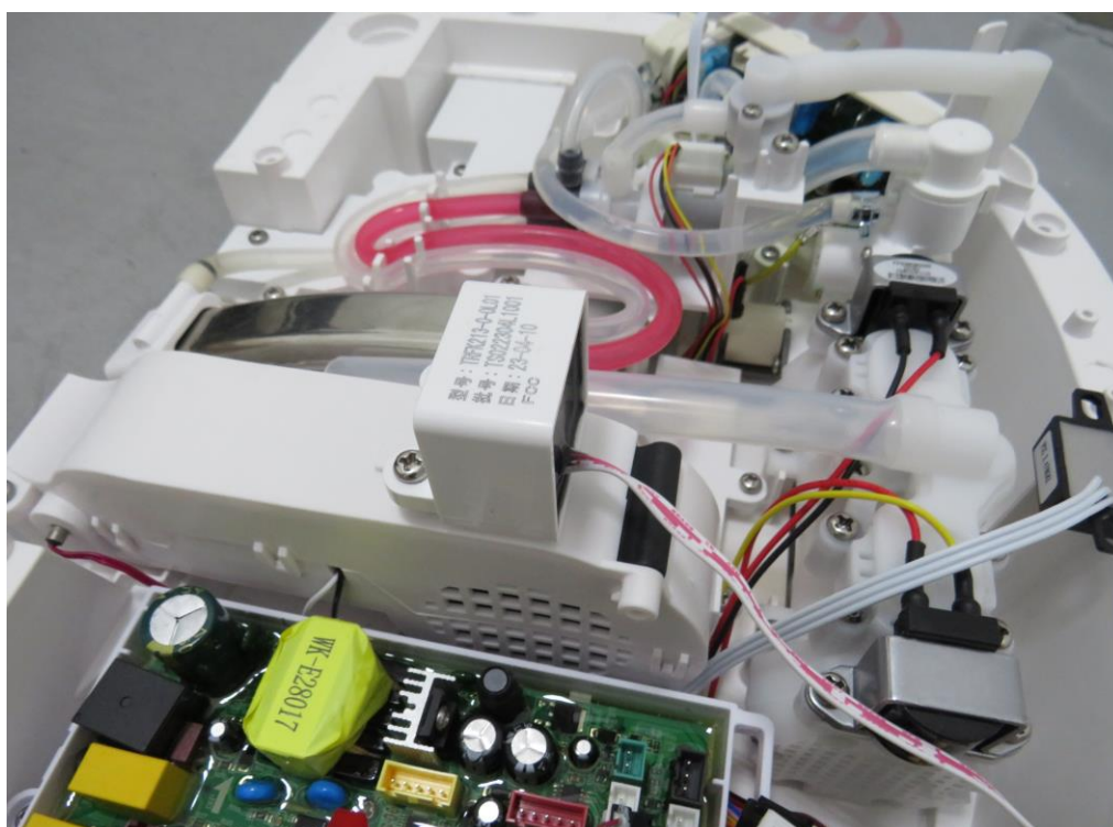
(12) EUT Photo
