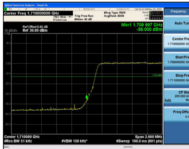
Band4-3MHz-QPSK-19965-1RB#14
