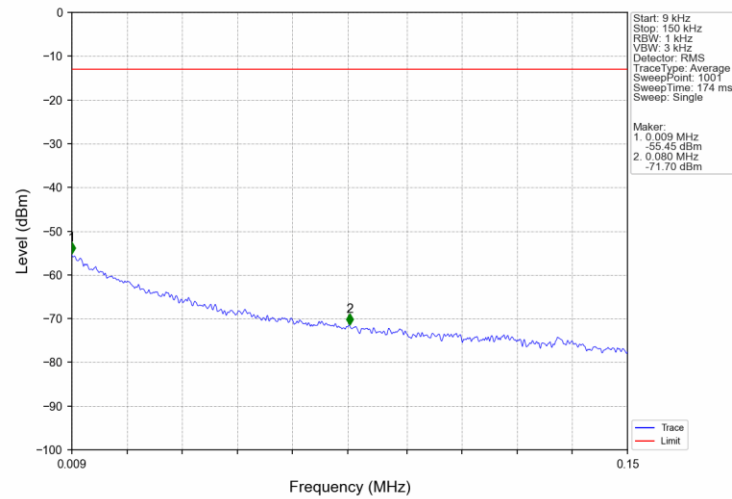
Band17 5MHz QPSK MCH 710MHz RB 1 0 NTNV
