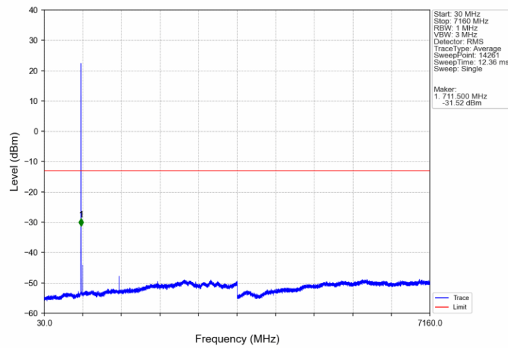
Band12 1.4MHz QPSK MCH 707.5MHz RB 1 0 NTNV
