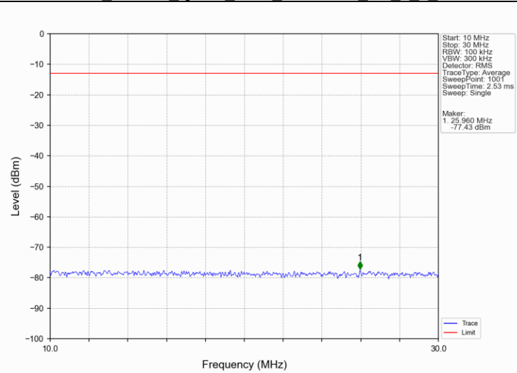
Band12 1.4MHz QPSK MCH 707.5MHz RB 1 0 NTNV
