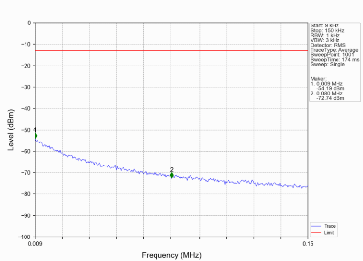
Band4 5MHz 16QAM LCH 1712.5MHz RB 1 0 NTV
