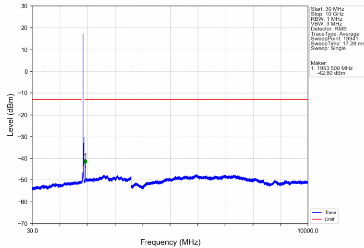
Band2 20MHz QPSK MCH 1880MHz RB 1 0 NTNV
