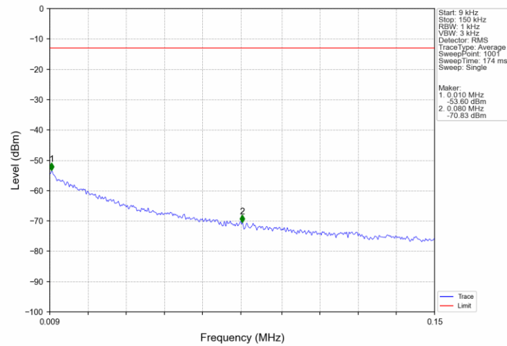
Band2_3MHz_16QAM_MCH_1880MHz_RB_1_0_NTNV
