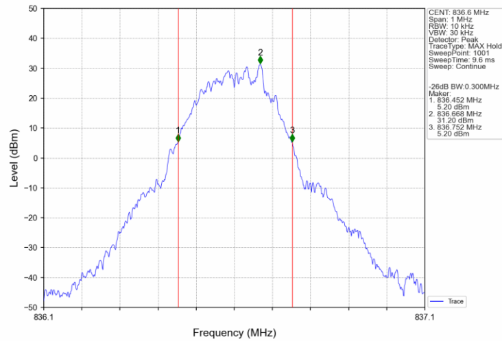
GSM850 GSM MCH 836.6MHz GSM_NTNV
