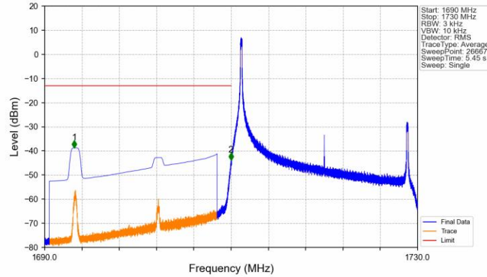
Band4_20MHz_QPSK_LCH_1720MHz_RB_1_0_NTNV
