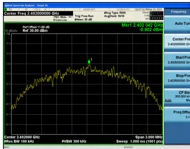
BLE_2M-Ant1-2402-30~1000--0.90
