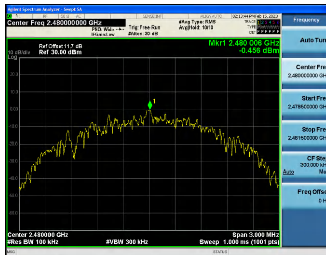
BLE_2M-Ant1-2480-30~1000--0.46
