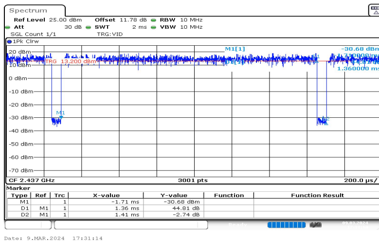
NTNV-11G-Ant1-2437
