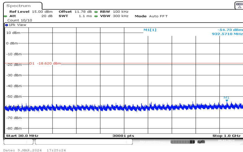
11G-Ant1-2412-30~1000-1.38
