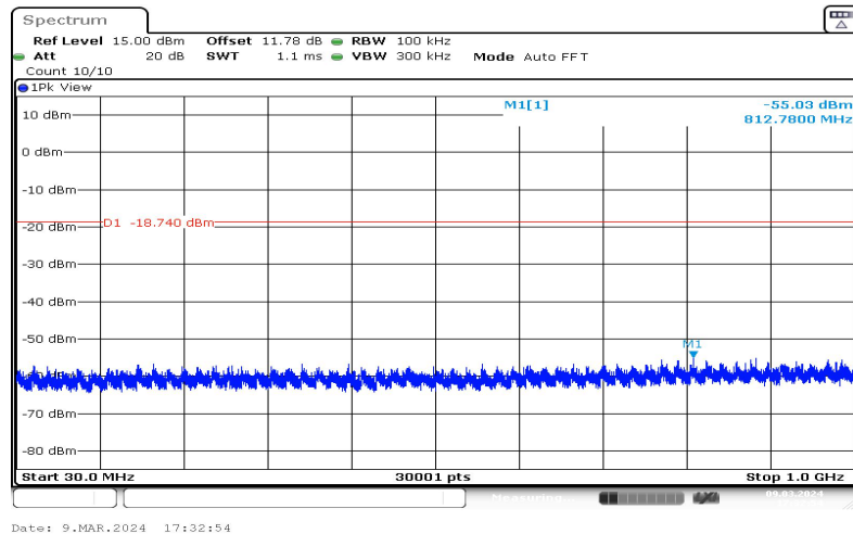
11G-Ant1-2437-30~1000-1.26
