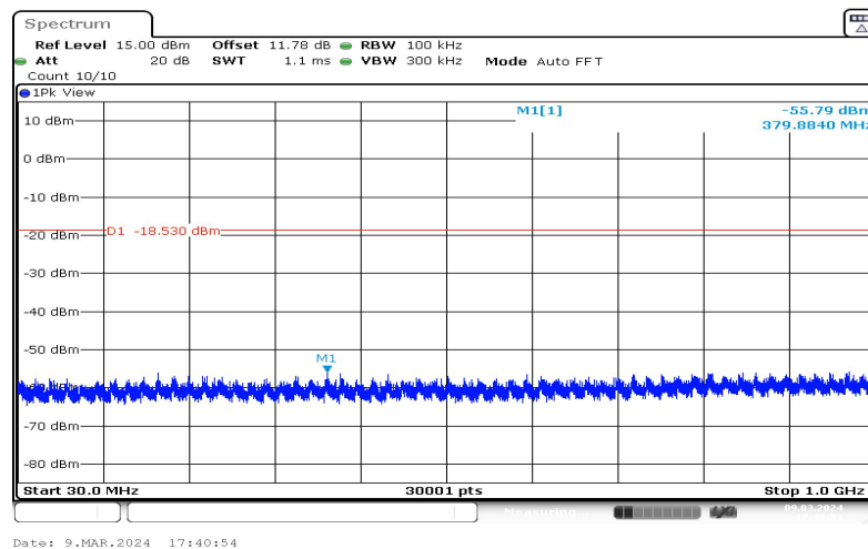
11N20SISO-Ant1-2412-30~1000-1.47
