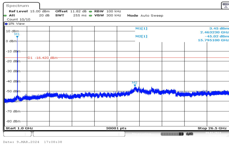
11B-Ant1-2462-1000~26500-3.58
