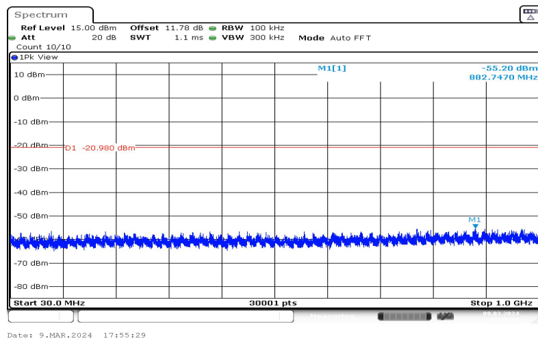
11N40SISO-Ant1-2422-30~1000--0.98
