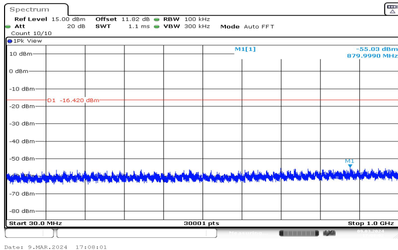
11B-Ant1-2462-30~1000-3.58
