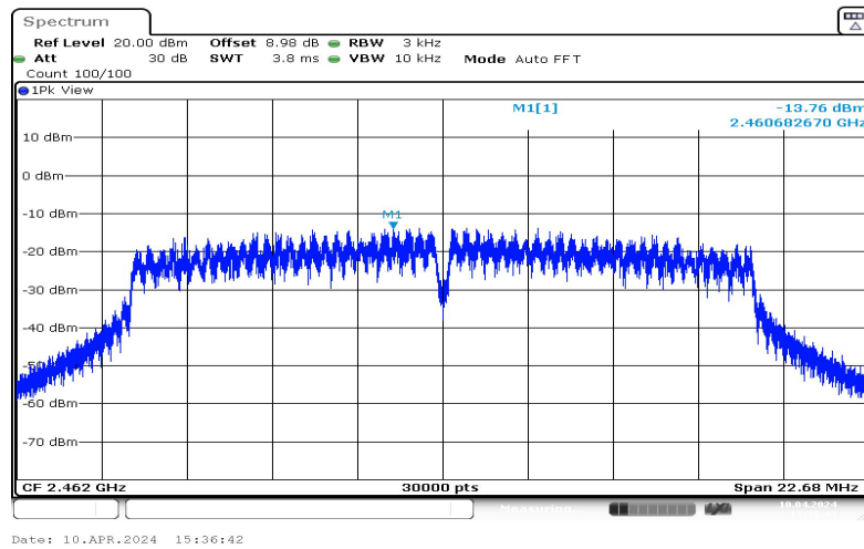
11G-Ant1-2462--13.76-0.00-0.00-0.00
