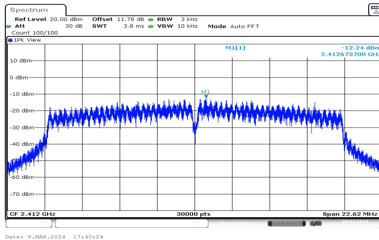
11N20SISO-Ant1-2412--12.24-0.00-0.00-0.00
