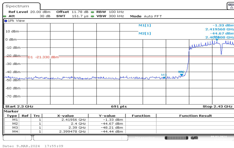
11N40SISO-Ant1-Low-2422--1.33
