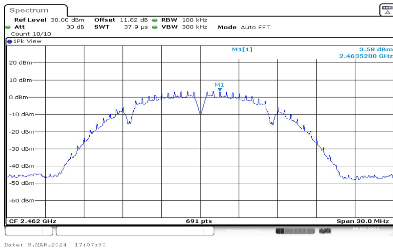
11B-Ant1-2462-0~Reference-3.58
