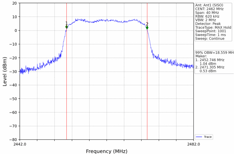
802.11n(HT20)_HCH_2462MHz_Ant1 (SISO)_NTNV
