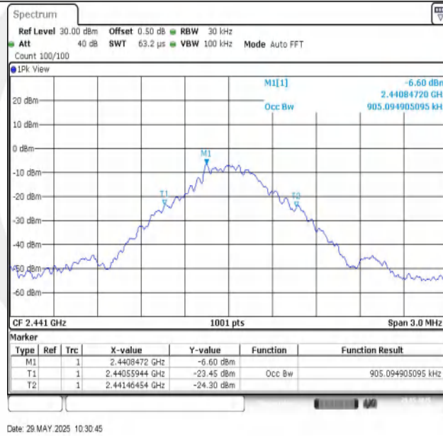
DH5-Ant1-2441
