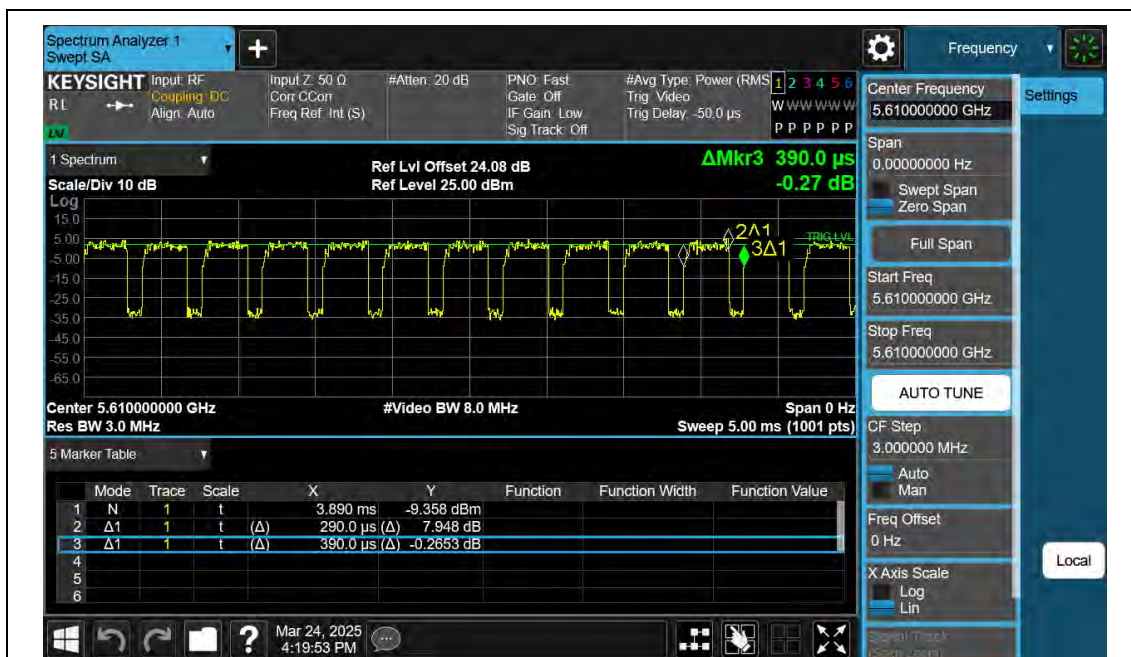
NTNV-11AX80SISO-Ant2-5610
