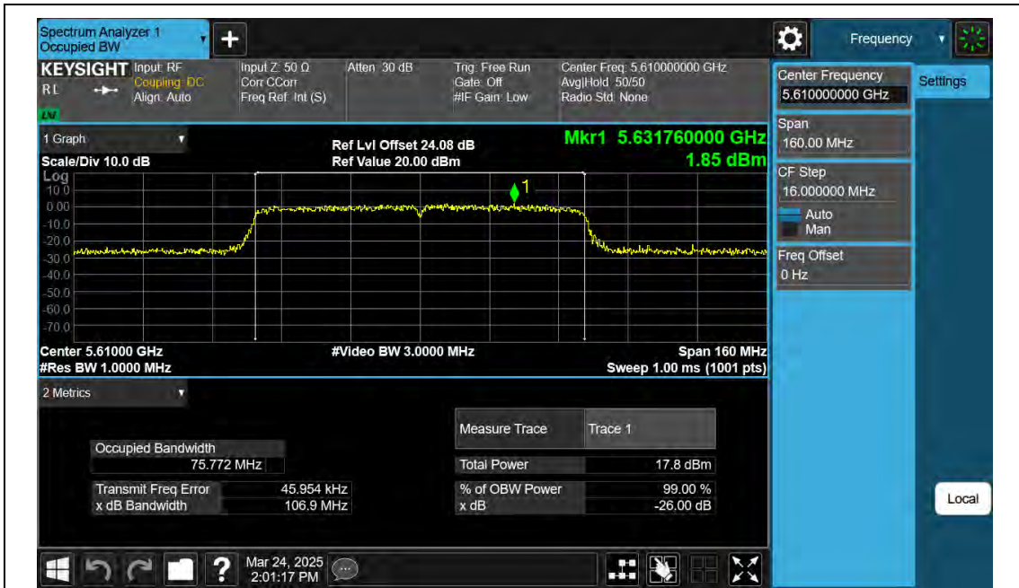
11AC80SISO-Ant2-5610
