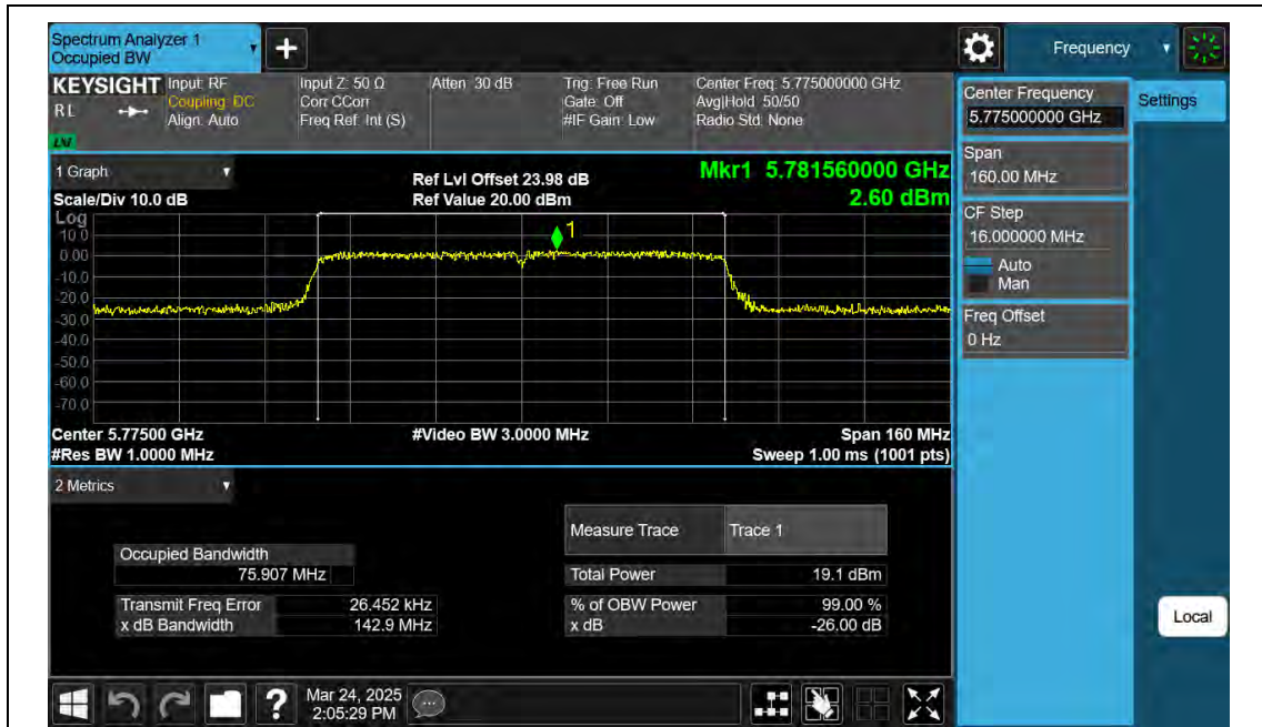
11AC80SISO-Ant2-5775
